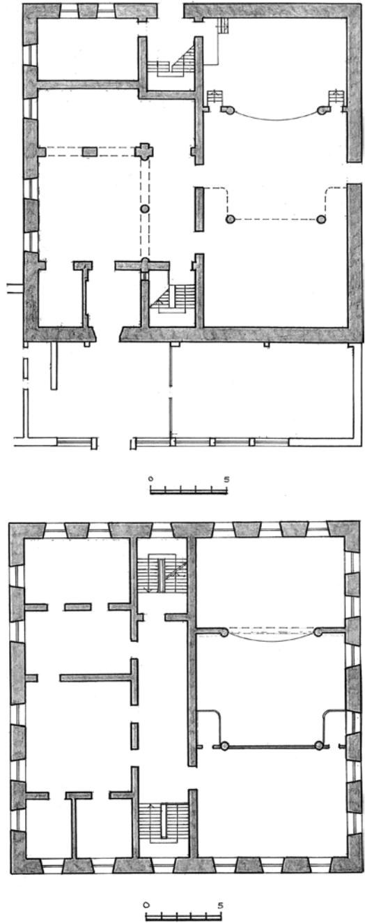
9 pav. Kupiškio Didžioji sinagoga: a – 1-ojo aukšto planas, b – 2-ojo aukšto planas. Sudarė A. Rupeika
