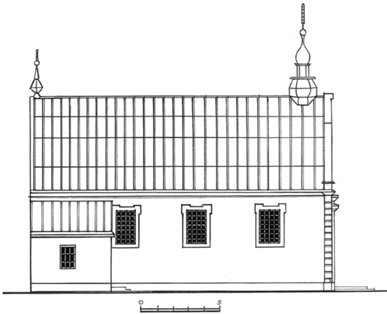
18 pav. Palėvenėlės bažnyčia: c – šoninis fasadas. KTU ASI
