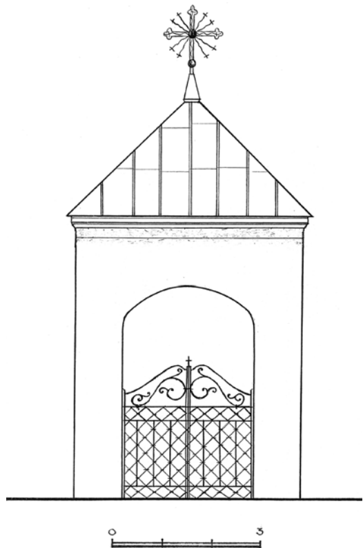
19 pav. Palėvenėlės vartai-varpinė: a – planas. Sudarė A. Rupeika; b – pagrindinis fasadas. KTU ASI
