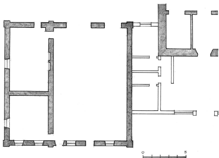
10 pav. Kupiškio chasidų sinagogos planas. Sudarė A. Rupeika
