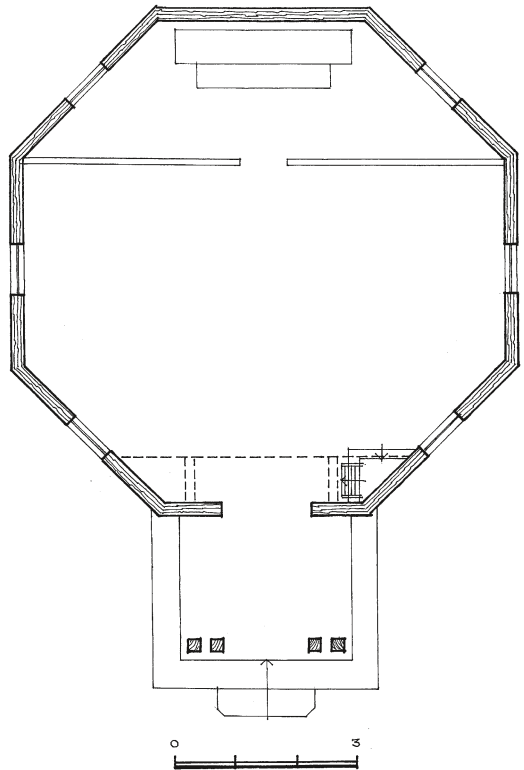
21 pav. Uoginių kapinių koplyčios planas. Sudarė A. Rupeika
