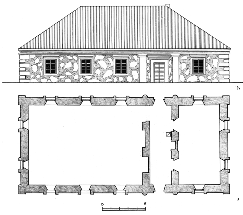
6 pav. Kupiškio parapijos mokykla (dab. muziejus): a – planas, b – pagrindinis fasadas. KTU ASI
