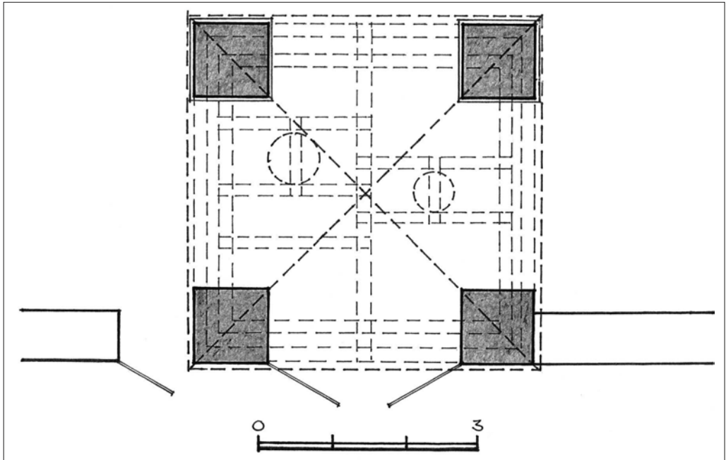
19 pav. Palėvenėlės vartai-varpinė: a – planas. Sudarė A. Rupeika; b – pagrindinis fasadas. KTU ASI
