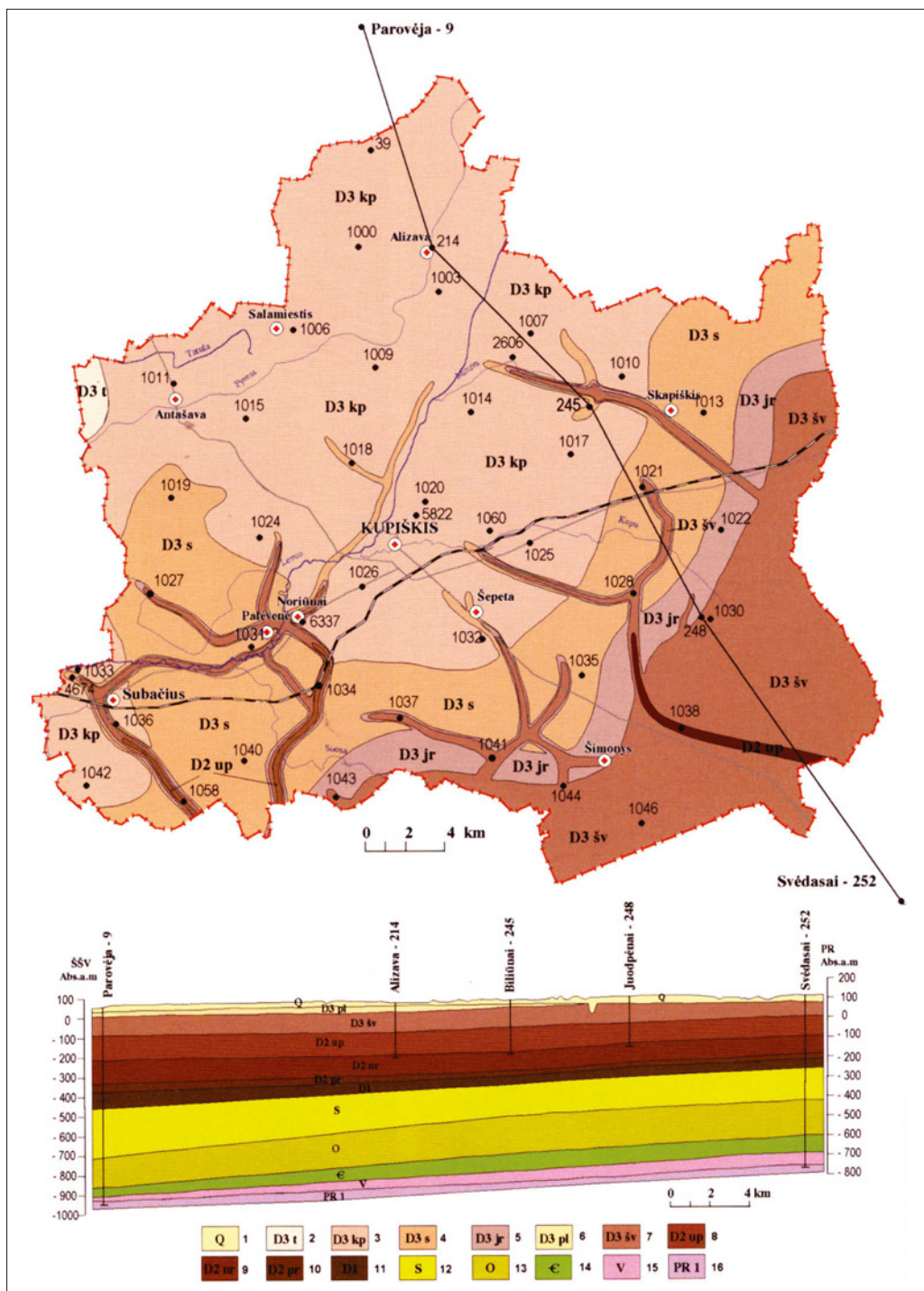
3 pav. Kupiškio r. prekvartero geologinis žemėlapis ir geologinis pjūvis: 1 – kvarteras; viršutinio devono svitos: 2 – Tatulos; 3 – Kupiškio; 4 – Suosos; 5 – Jaros; 6 – Plevinių regioninis aukštas; 7 – Šventosios; 8 – Upininkų serija; 9 – Narvos serija; 10 – Pernu svita; 11 – apatinis devonas; 12 – silūras; 13 – ordovikas; 14 – kambras; 15 – viršutinis proterozojus (vendas); 16 – apatinis proterozojus. Iš V. Marcinkevičiaus str. Geologinė apžvalga, Kupiškėnų enciklopedija, V., 2006, t. 1
